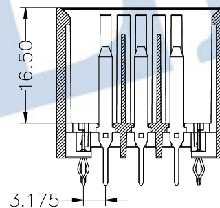
A-A SECTION
