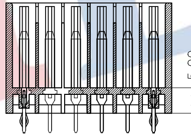
A-A SECTION
