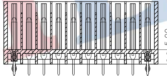
A-A SECTION
